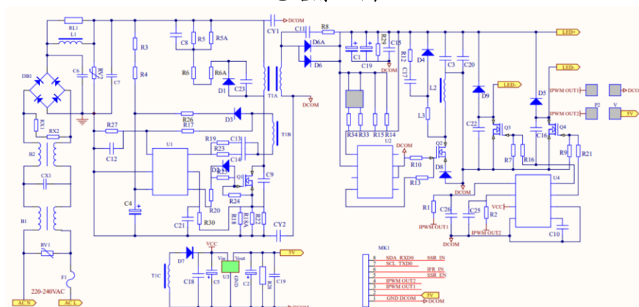
电路原理图
