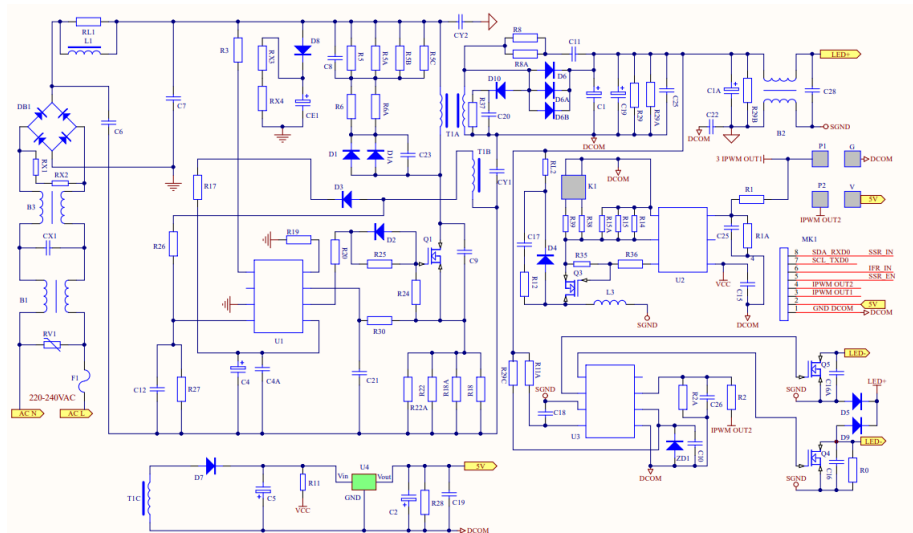
电路原理图
